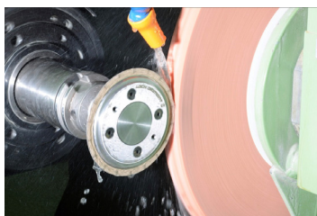
drebojet®-plus-Form-Abrichtrolle
